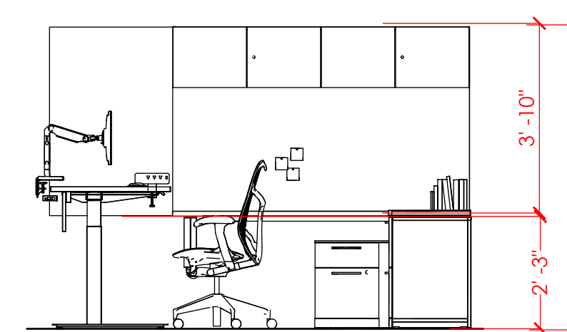
Elevation B
