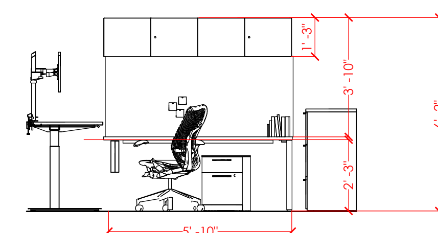
Elevation A
